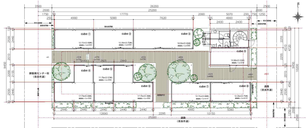
1階平面図・配置図
