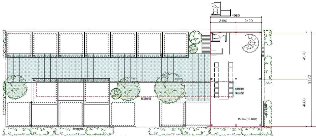
2階平面図
